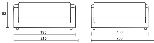
Divano letto con 2 tipi di braccioli
