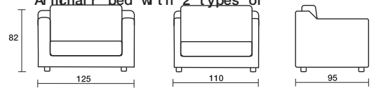
Poltrona letto con 2 tipi di braccioli Armchair bed with 2 types of
